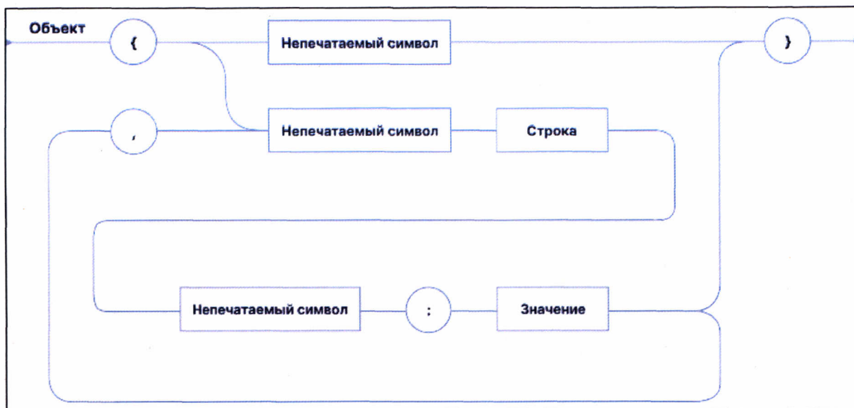
Рис. 9.1. Схема синтаксиса объекта
