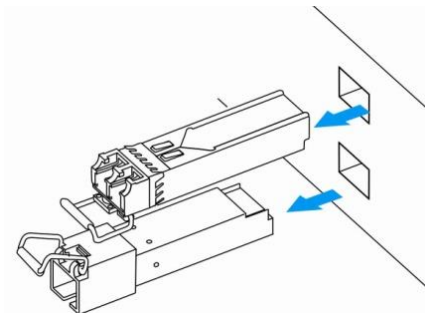
Рисунок 46 – Извлечение SFP-трансиверов
