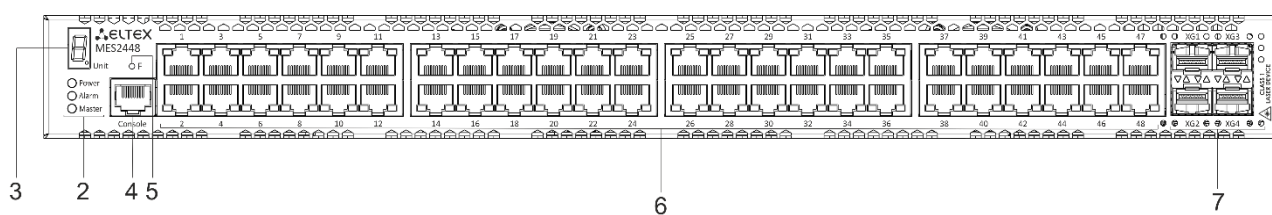
Рисунок 20 – Передняя панель MES2448 DC
